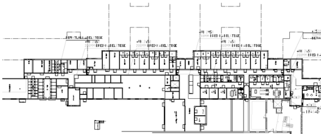
Kabeldragningen
